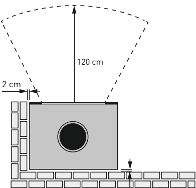
Draufsicht Brennkammer
