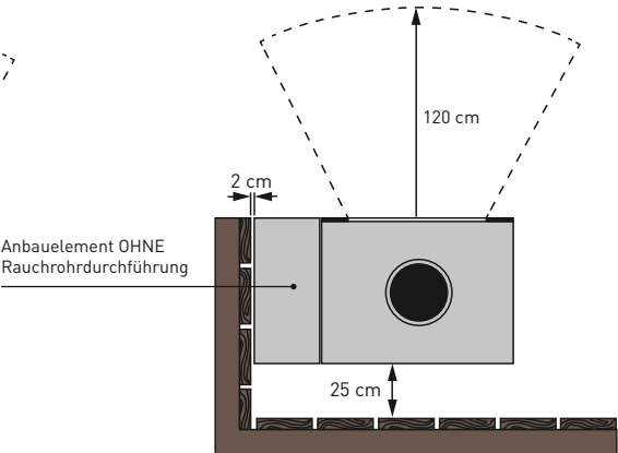
Draufsicht Brennkammer
