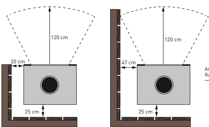
Draufsicht Brennkammer
