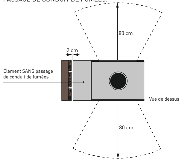
B CHAMBRE DE COMBUSTION AVEC ÉLÉMENTS LATÉRAUX SANS PASSAGE DE CONDUIT DE FUMÉES:
