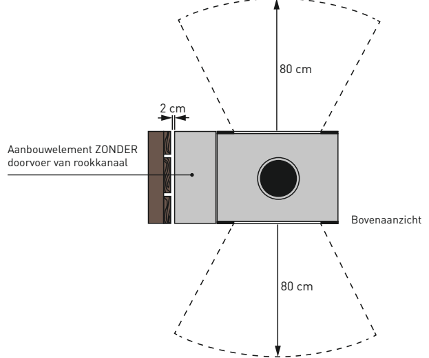
B VERBRANDINGSKAMER MET ZIJDELINGSE AANBOUWELEMENTEN ZONDER DOORVOER VAN ROOKKANAAL:
