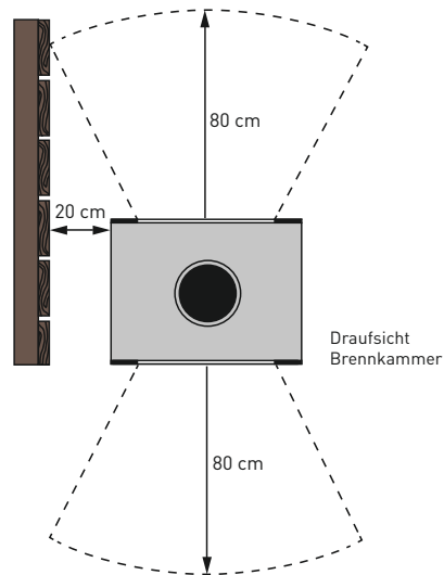
A BRENNKAMMER OHNE SEITLICHE ANBAUELEMENTE:
