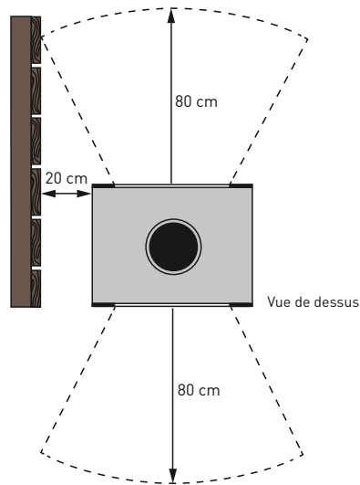
A CHAMBRE DE COMBUSTION SANS ÉLÉMENTS LATÉRAUX:
